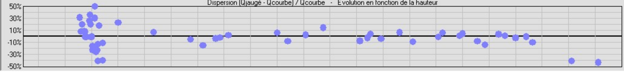
Dispersion (Qjaugé - Qcourbe) / Qcourbe - Evolution en fonction de la hauteur
