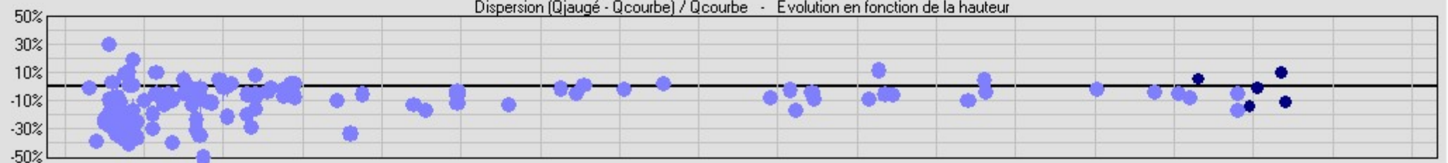
Dispersion (Q_{\text{jauge}} - Q_{\text{courbe}}) / Q_{\text{courbe}} - Evolution en fonction de la hauteur
